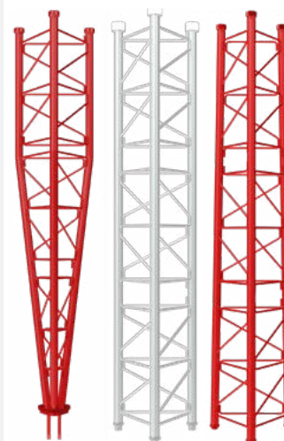
▲ Tramos 550
